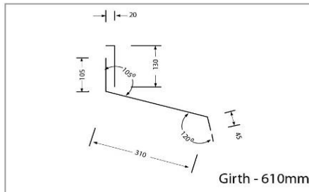
APRON FLASHING
